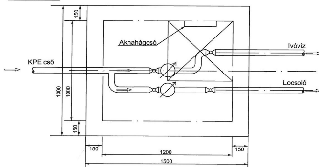
Felülnézet
